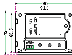
底视图 Bottom view
